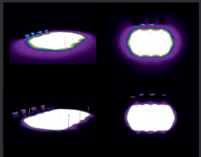
Zintegrowane rozwiązanie oświetlenia LT, LTM i LO przeznaczone do asymetrycznej wiązki światła
